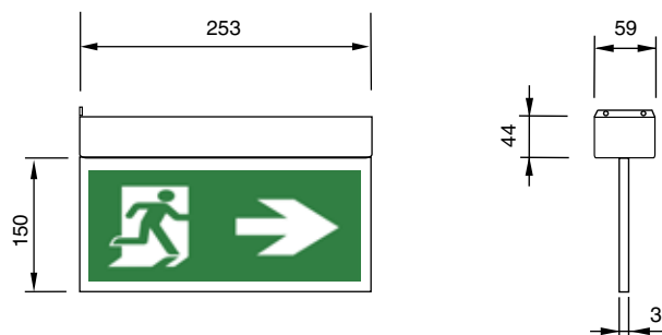
Banderola
