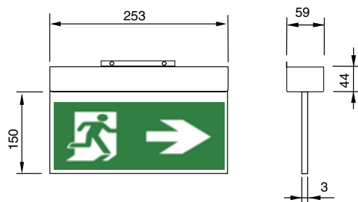
Banderola
