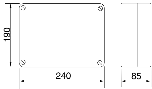
Cuadro Centralizado
