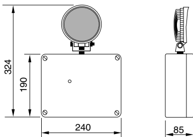
Un Foco
