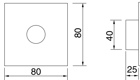
Cuadrada
