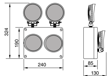
Cuatro Focos
