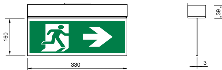
Banderola
